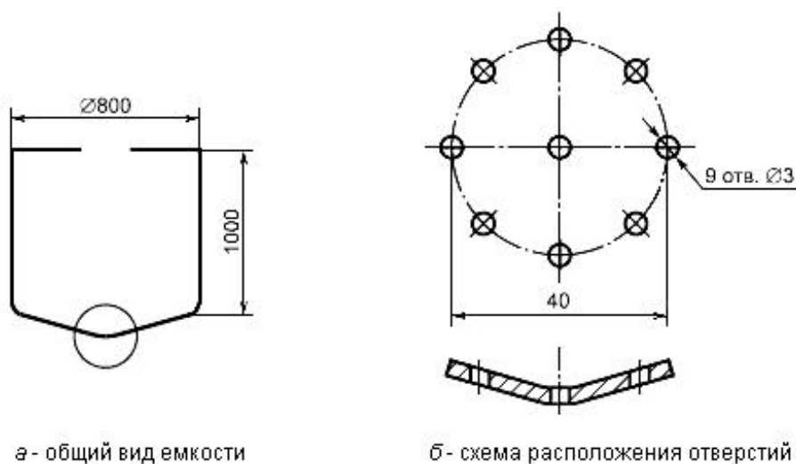
Рисунок 5 - Емкость для сбора пены
