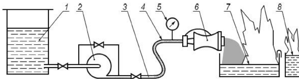
Рисунок 7 - Схема установки для тушения пеной средней кратности
